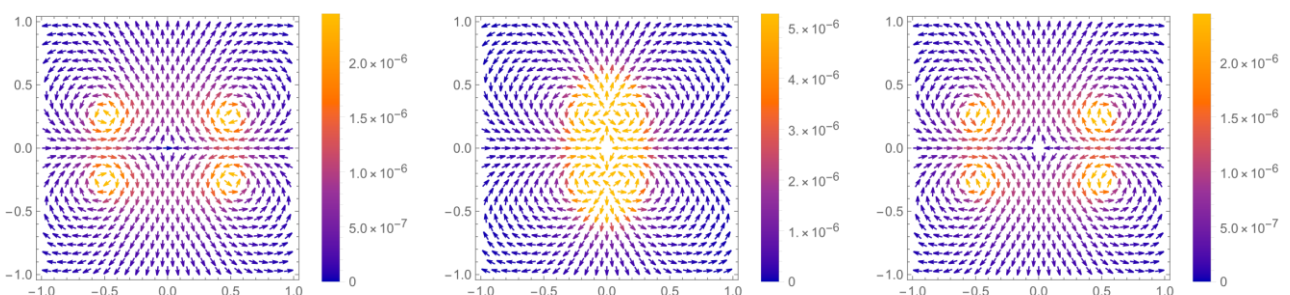
Figura 2: campo de una espira (dipolo) con la ley de Biot-Savart, con la aproximación dipolar y con cálculo directo mediante funciones elípticas.
