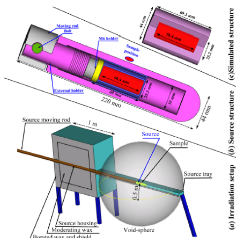
Figura 1. Ejemplo de un contenedor para una muestra de AmBe [1].
